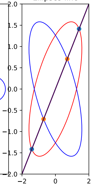
Ellipses-line
